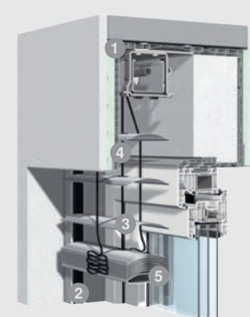
Unterputzausführung
